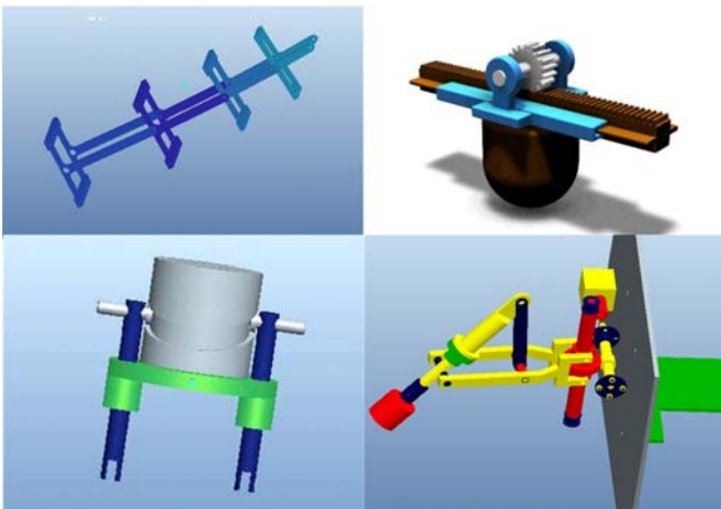
图1 机器海豚分功能原理求解
