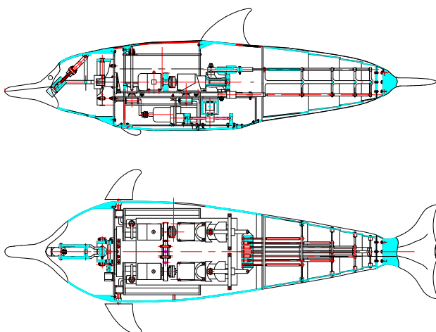
图2 机器海豚分功能原理解组合设计方案
